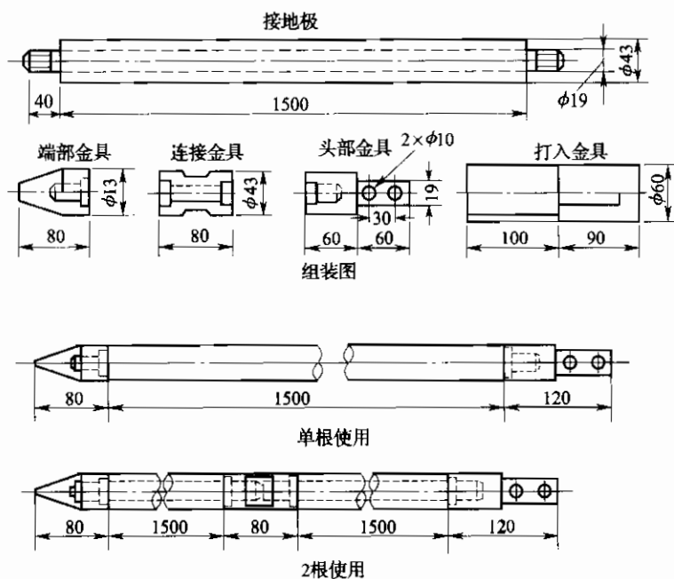
图 2 锌接地极结构图
