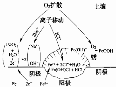
图 1 氧浓差电池的腐蚀模型
